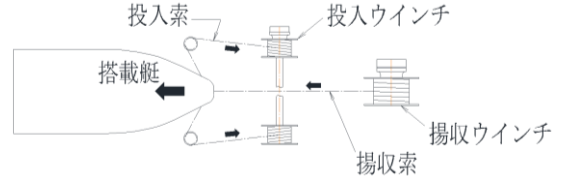
図2 投入ウインチ Fig.2 Launch winch
