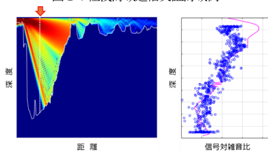
図2：音響伝搬解析例
